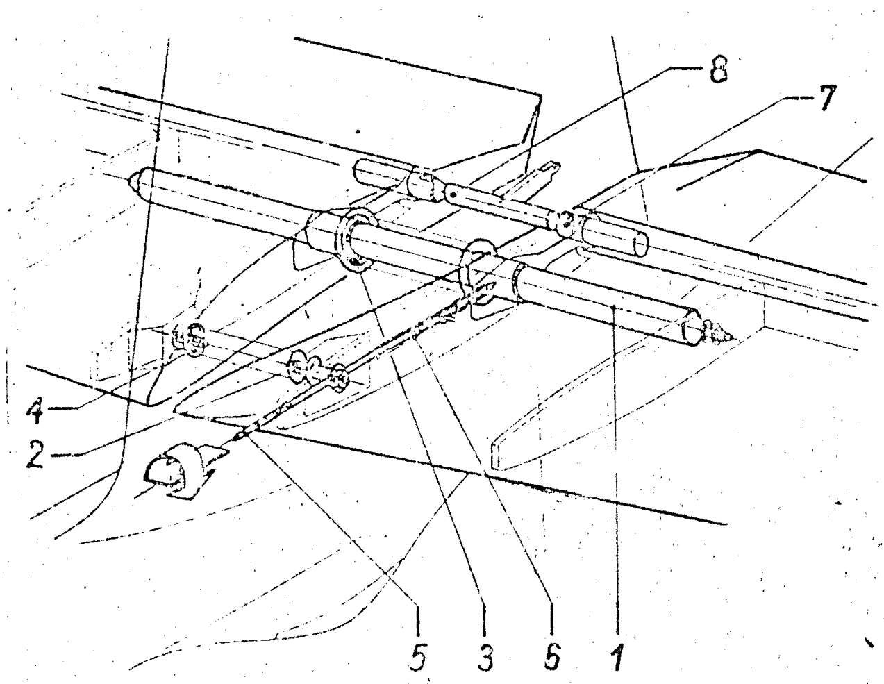
Rys. 7: Montaż ustzerzenia wysokości
