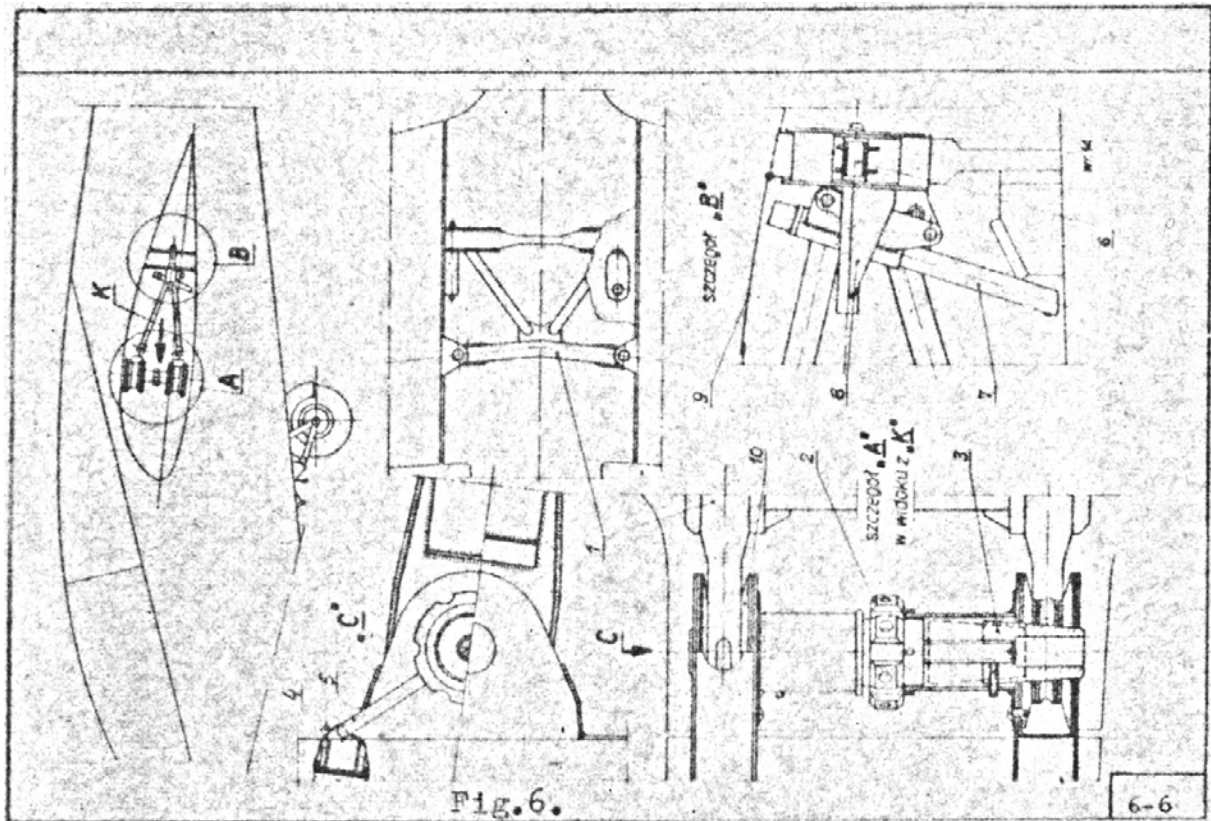
Fig.6 Montaż skrzydła
