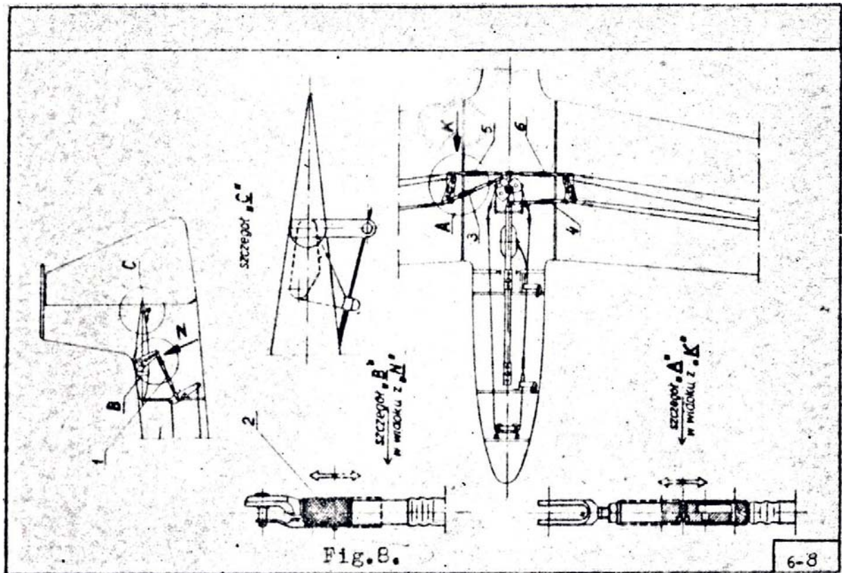
Fig.8 Połączenie napędów steru wysokości
